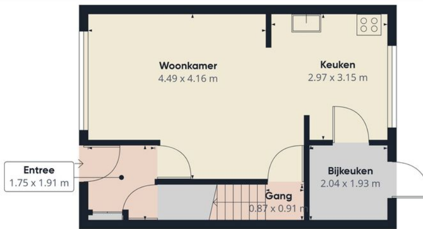
Etage 0
